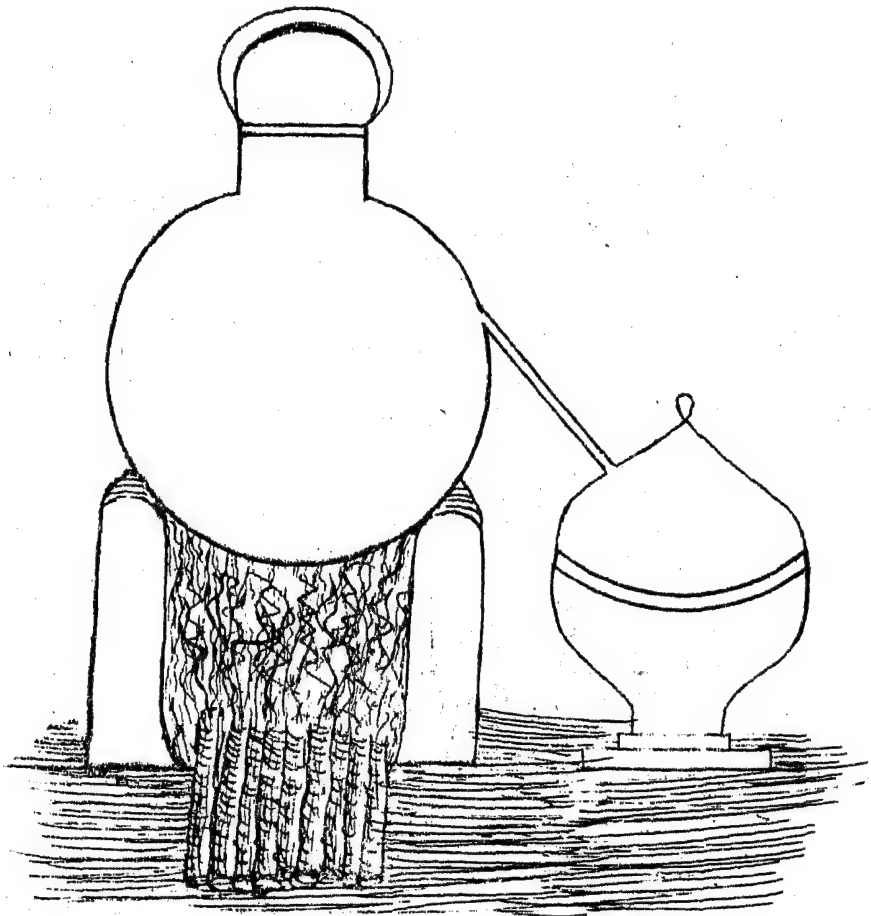
ढकीयन्त्रम् ६
